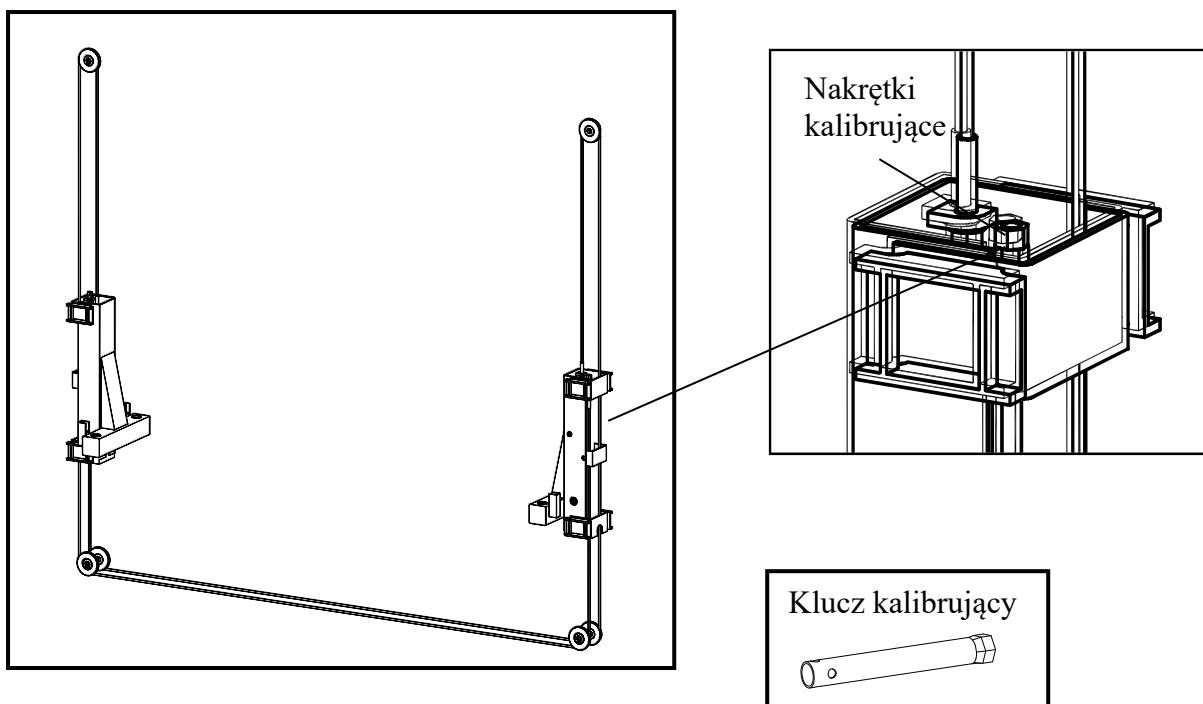
Rysunek 11 – PROWADZENIE PRZEWODÓW WYRÓWNAWCZYCH
