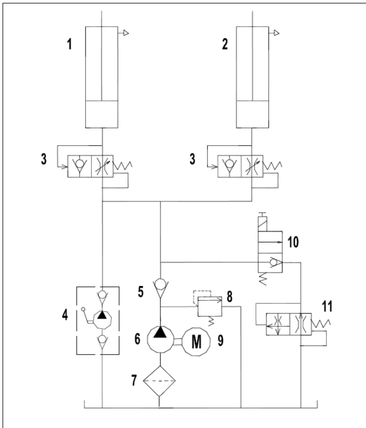
Rysunek 5 - SCHEMAT HYDRAULICZNY
