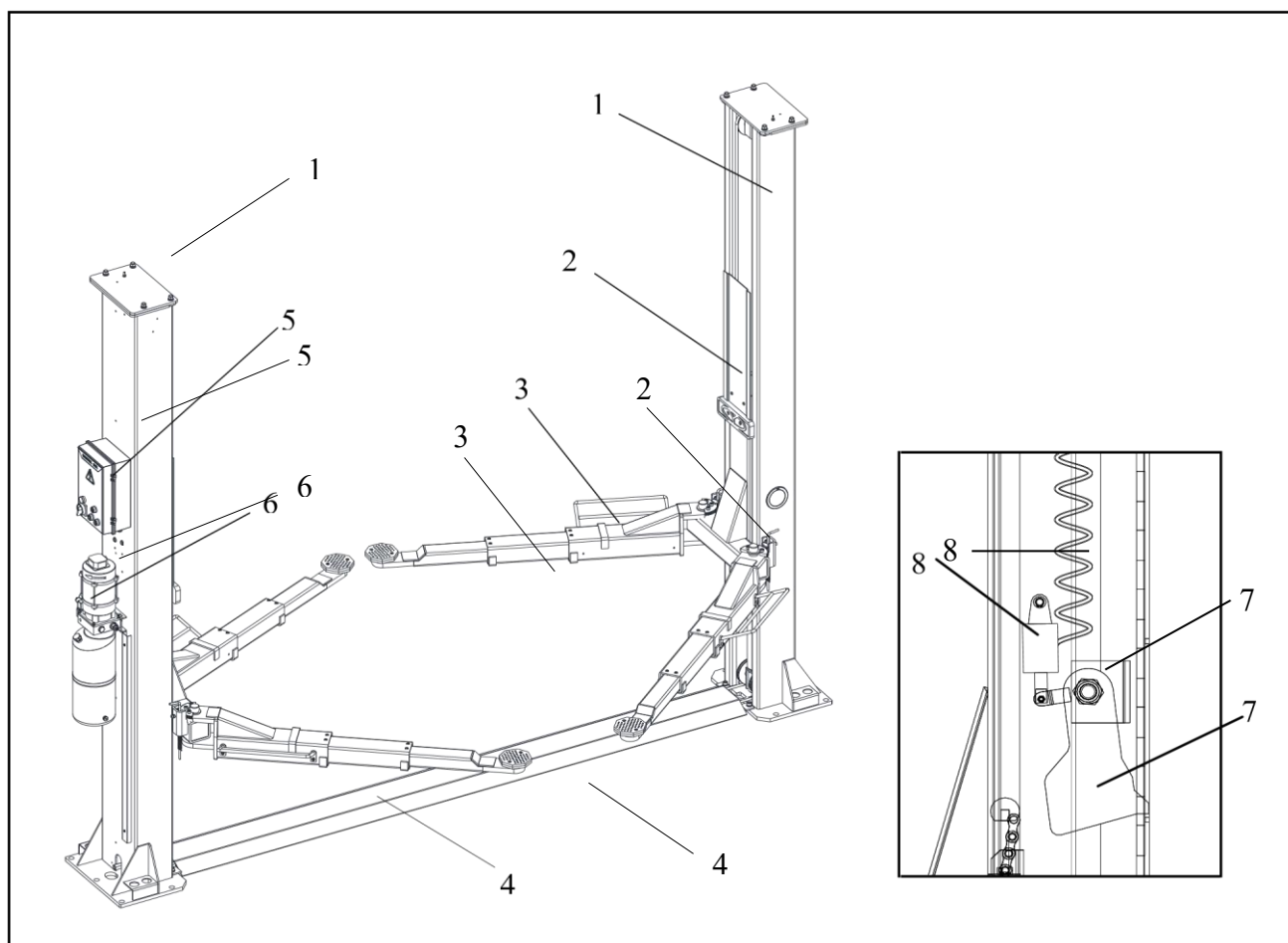
Rysunek 2 – PODNOŚNIK
